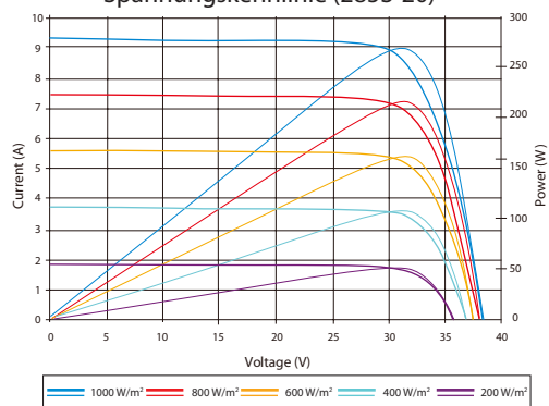
Strom-Spannungs- & Leistungs-Spannungskennlinie (285S-20)
